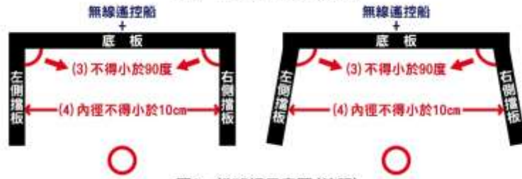
圖2、推球板示意圖(俯視)
